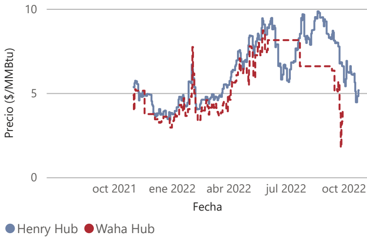
Precios de combustibles [$/MMBtu]
