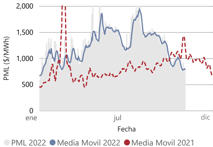
PML (históricos) [$/MWh]
