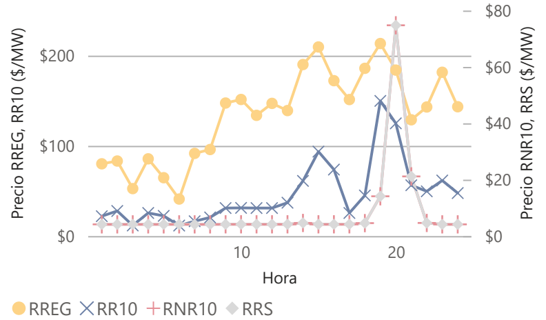
Precios de Servicios Conexos [$/MW]†
