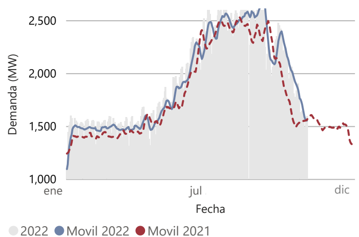
Demanda (históricos) [MW]
