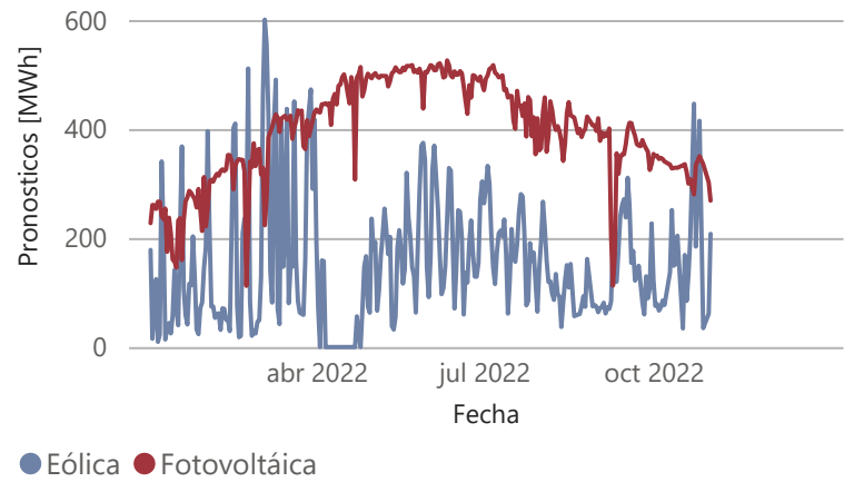
Pronósticos de generación RN [MWh]
