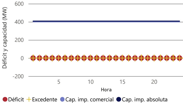
Déficit, excedentes, y capacidad de transferencia de importación [MW]
