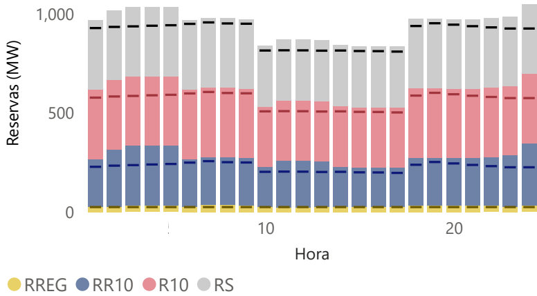
Asignación y requerimientos de Servicios Conexos [MW]†
